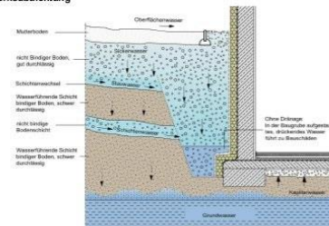
Bauwerksabdichtung
